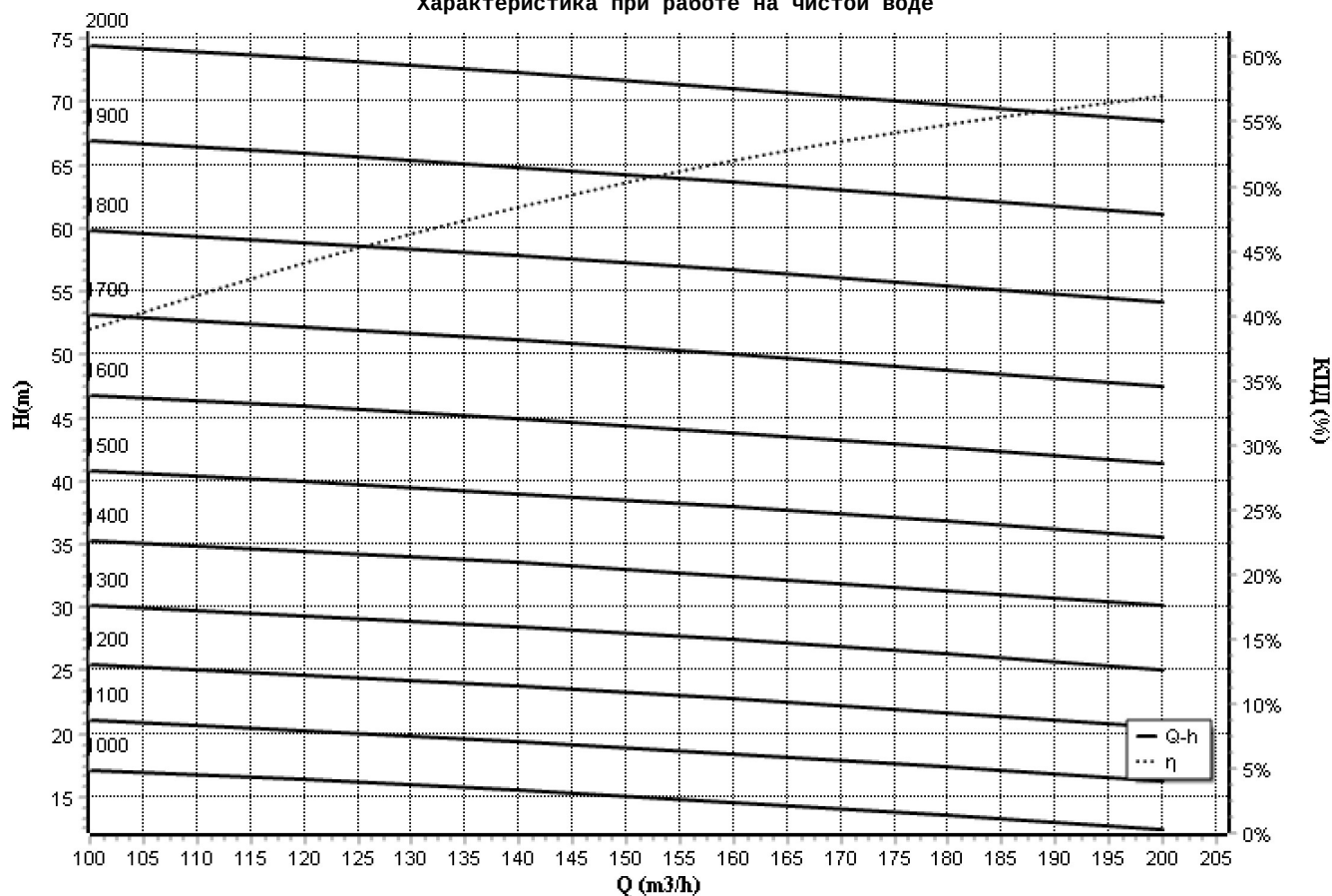
Характеристика при работе на чистой воде
